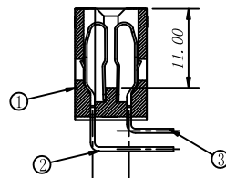
剖视图 A-A
