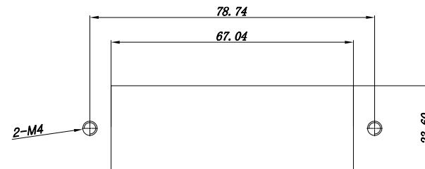
推荐PCB开板尺寸 (公差±0.05mm)
