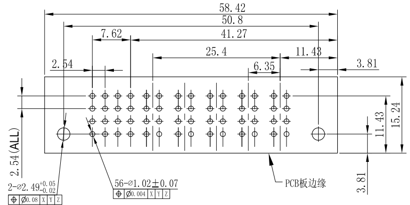
PCB开孔尺寸 连接器装配方向
