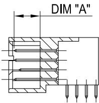
剖面 A-A
