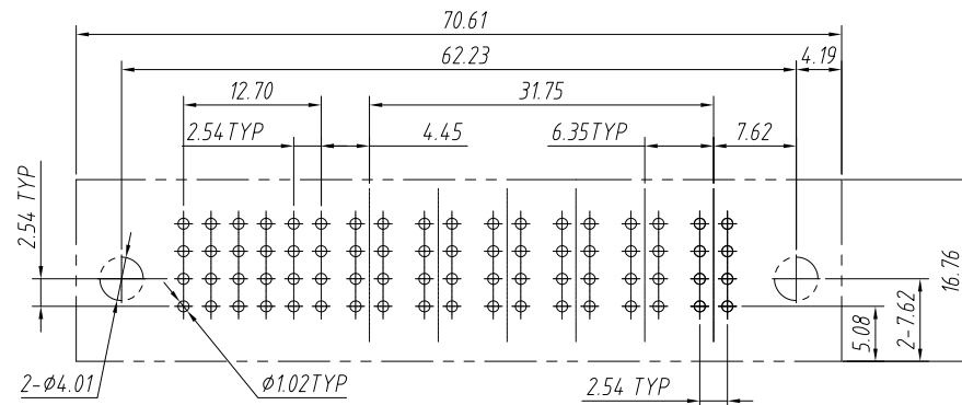
推荐PCB开孔尺寸( \pm 0.05 )
