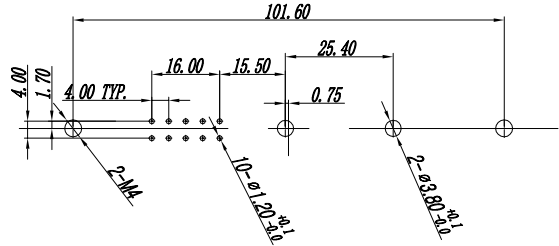
推荐PCB板开孔尺寸 (公差±0.05mm)
