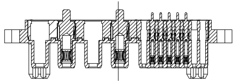
截面A-A
