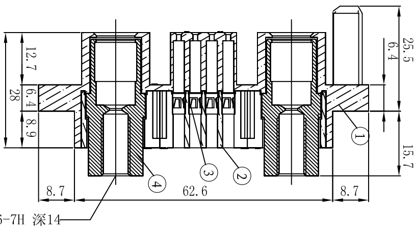
剖面 A-A
