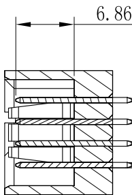
剖视图 A-A
