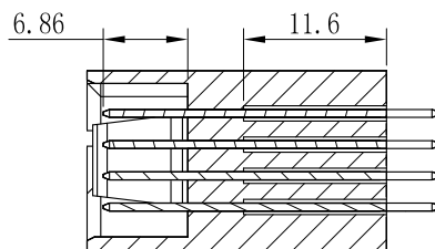
剖视图 A-A
