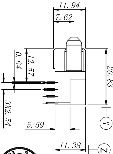
剖视图 B-B
