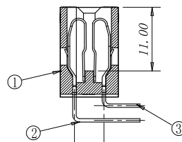
剖视图 A-A
