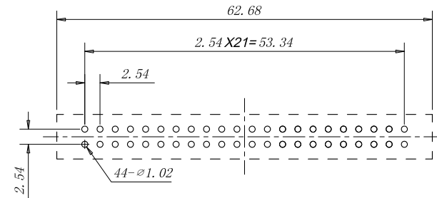
推荐PCB板布局
