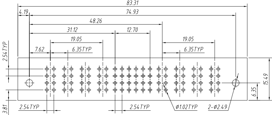
推荐PCB开孔尺寸(公差±0.05)
