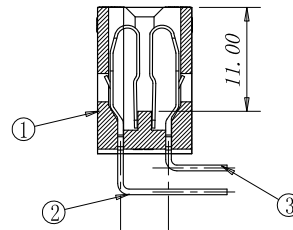
剖视图 A-A
